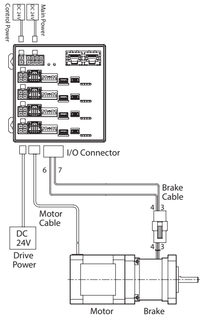
Ezi-STEPII EtherCAT 4X
